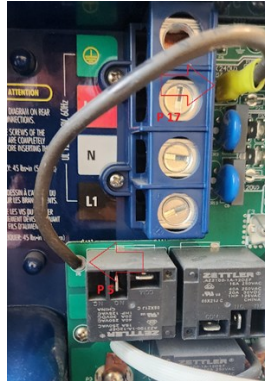
FIGURE 2: 240 VOLT CONFIGURATION
